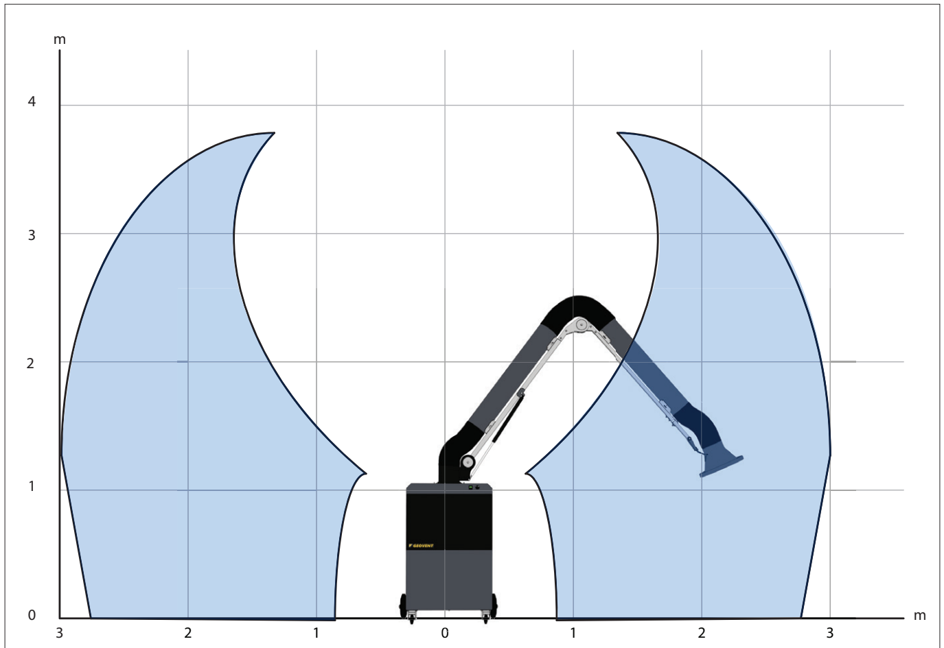
Arbeitsbereich des GeoGo Black W3 mit 3m ASA4 Arm
