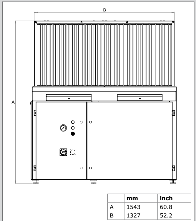
Absaugtisch mit BackDraft Kit (Vorderseite)
