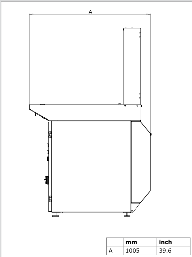
Absaugtisch mit BackDraft Kit (Seitenansicht)
